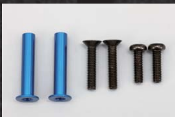
ステアリング ベルクランク ポスト (軽量アルミ製)
