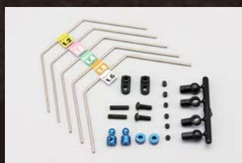
フロント スタビ セット (5 種類入) (深リム仕様を除く)
