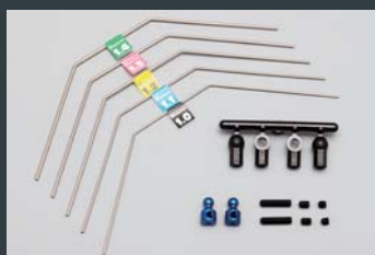
スタビ セット
