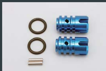
センタードライブ カップ (アルミ製) SD-644A ¥1,800 センターシャフトの回転精度を上げるアルミ削り出しカップ。
