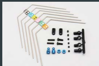
リア スタビ セット (6 種類入) (深リム仕様を除く) SD-412RS ¥1,380 ドリフト中のリアの引っ掛かりを防ぐスタビライザーのセット。ワイヤー 6 種入り。
