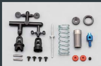
フロント ショック セット (ワイド仕様・1本入)
