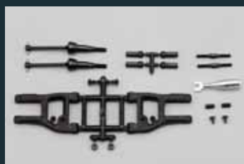
深リムホイール専用 リヤサスペンション セット (φ2ピン仕様 ユニバーサル)
