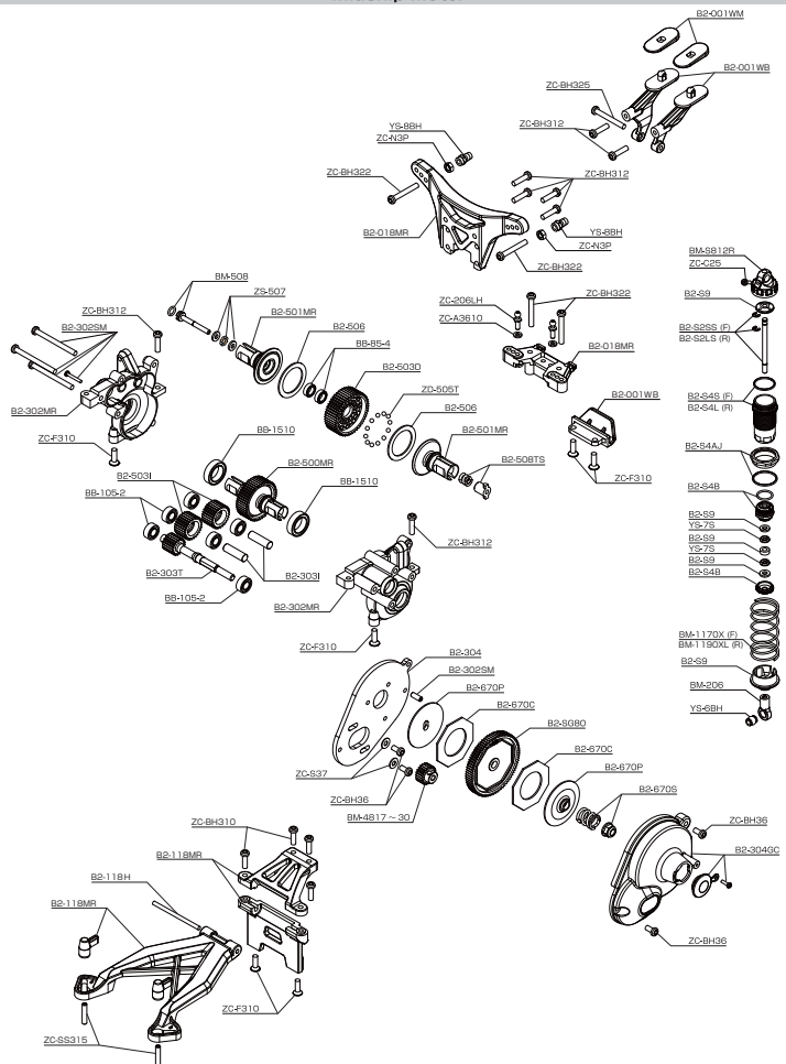
●ミッドシップ モーター● Midship Motor
