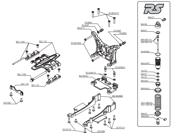
●リヤモーター● Rear Motor
