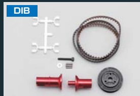
DIB フルカウンター ソリッドアクスル セット (リヤ 1.5 倍 ブルー/レッド) IB-FCD15/15R 各 ¥3,750 フロント 1 回転に対し、リヤが 1.5 回転する FCD アクスル。FCD としては標準的な比率。
