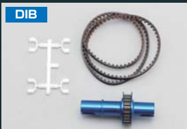
DIB フルカウンター ソリッドアクスル セット (リヤ 1.8 倍 ブルー/レッド) IB-FCD18/18R 各 ¥3,750 かなりアグレッシブな 1.8 倍の駆動比率。深いドリフトアングルやハイグリップ路面に対応。
