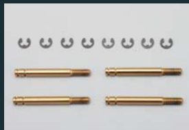
チタンコートショックシャフト (4 本入) YS-53S-4T ¥1,580 チタンコーティングを施しシャフトの傷を大幅に低減、ショック O リングの傷みを防止します。
