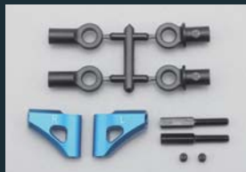
アルミ製 アッパー A アームセット (ブルー/レッド) D-140/140R 各 ¥3,200 フロント A アームキット用のアルミ A アームセット。キャンバーを無段階調整可能。
