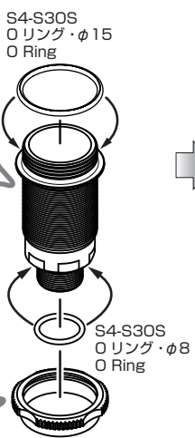
S4-S4M13 リアショックボディ・ショート Rear Shock Body · Short
