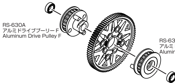
RS-630A アルミ F/R ドライブプーリー (20T) × 各 1 Aluminum F/R Drive Pulley ×1 Ea.
