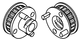
RS-630A アルミ F/R ドライブプーリー (20T) × 各 1 Aluminum F/R Drive Pulley ×1 Ea.
