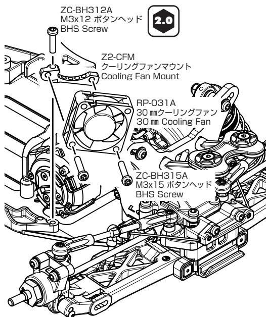
RP-031A 30mmクーリングファン ×1 30 mm Cooling Fan
