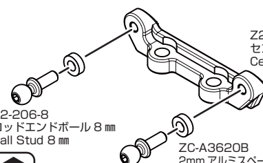
ZC-A3620B 2mm アルミスペーサー・黒 2mm Aluminum Spacer・Black
