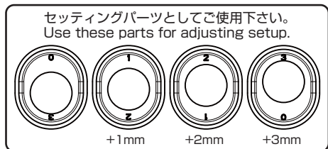
Z2-302CT ハイトアダプター 0/3 Height Adapter
